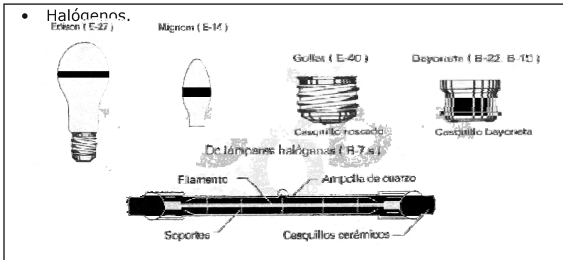
Tipos de casquillos
