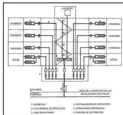
Instalación de enlace.
