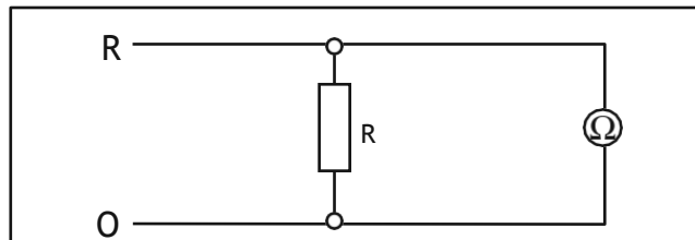
Colocación de un Óhmetro
