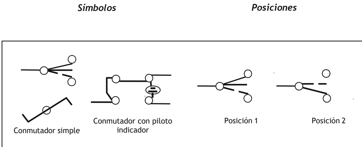
Símbolos empleados para los conmutadores
