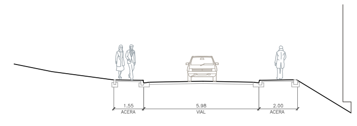
245 SECCION 5-5
