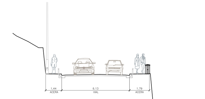
230 SECCION 2-2
