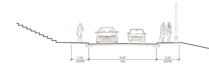
221 SECCION 1-1
