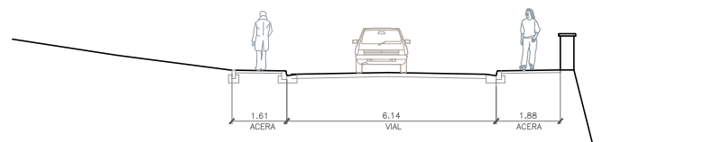
250 SECCION 6-6
