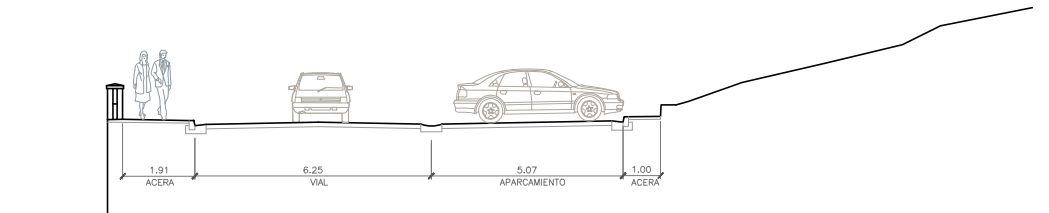
262 SECCION 9-9
