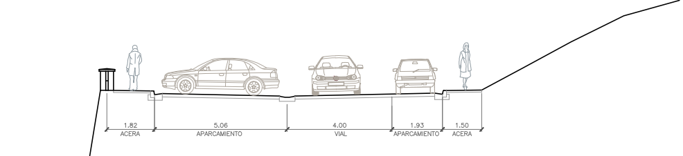
250 SECCION 7-7
