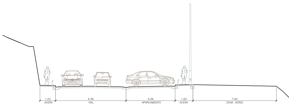
240 SECCION 4-4
