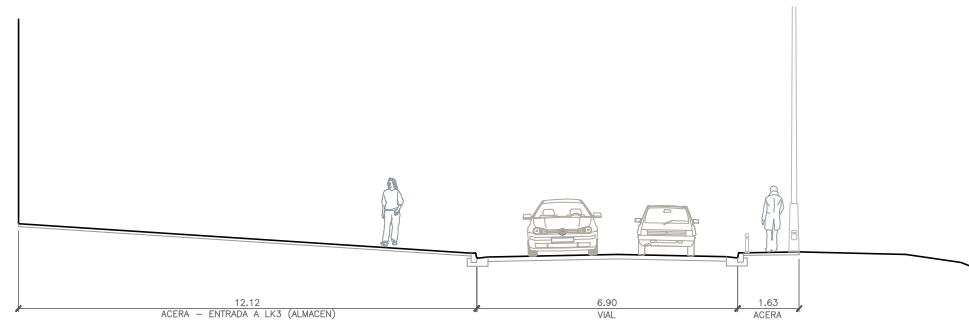
SECCION 12-12
