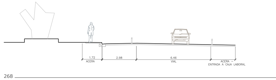
SECCION 14-14
