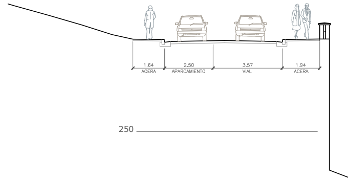
SECCION 17-17
