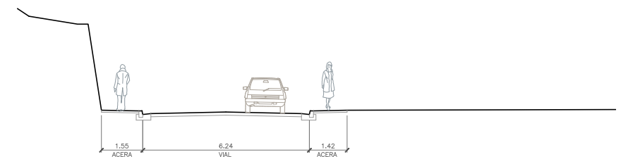
SECCION 19-19
