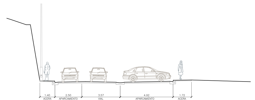
SECCION 19-19
