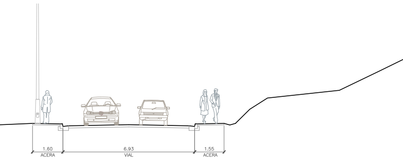
SECCION 14-14
