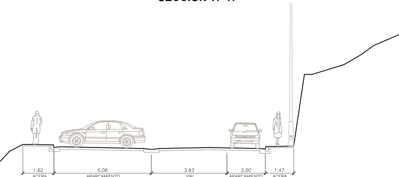
SECCION 17-17
