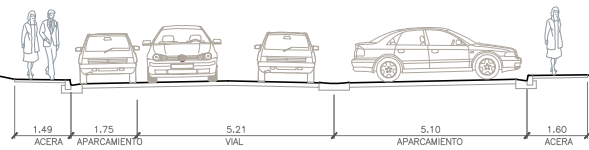
SECCION 13-13
