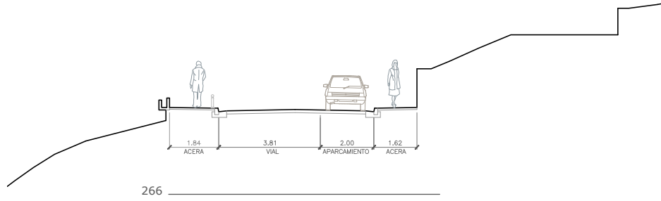
SECCION 15-15
