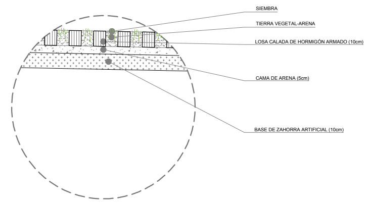
DETALLE NUEVO PAVICESPED SOBRE AGOMERADO EXISTENTE E=1/25
