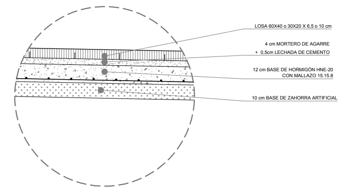
DETALLE NUEVA ACERA SOBRE ACERA EXISTENTE E=1/25
