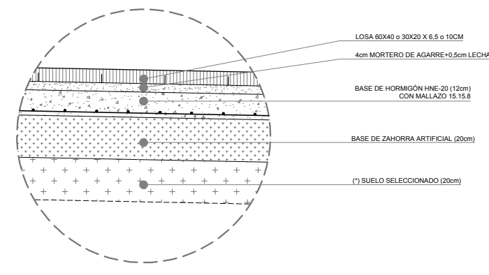
DETALLE NUEVA ACERA SOBRE ZONA VERDE E=1/25
