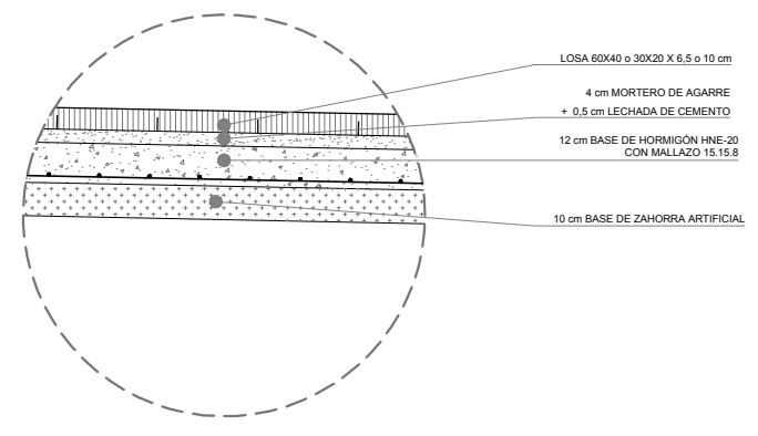
DETALLE NUEVA ACERA SOBRE ASFALTO EXISTENTE E=1/25
