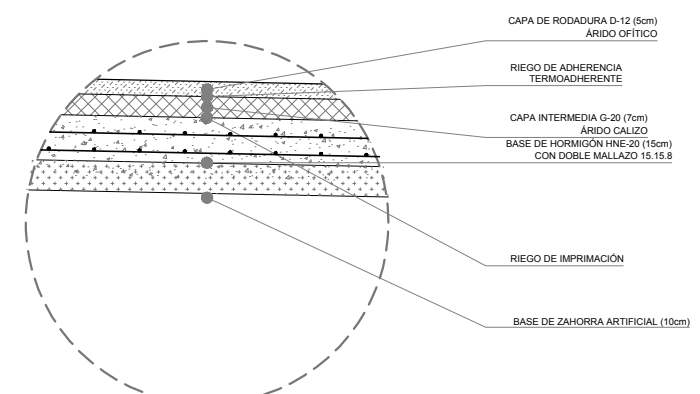
DETALLE NUEVO PARKING ASFALTO SOBRE ACERA EXISTENTE
