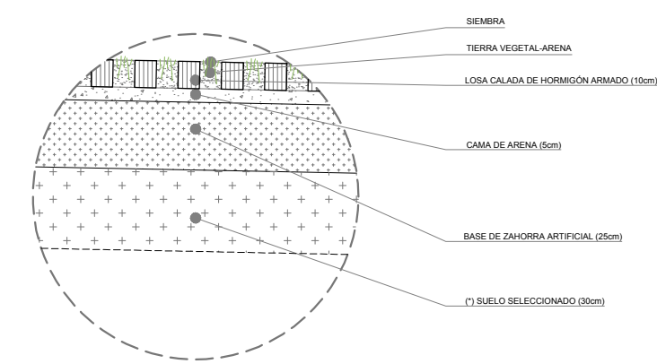
DETALLE NUEVO PAVICESPED SOBRE ACERA EXISTENTE
