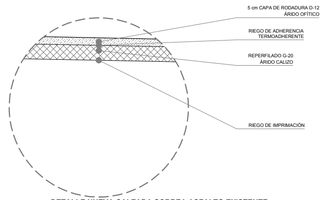
DETALLE NUEVA CALZADA SOBREA ASFALTO EXISTENTE E=1/25
