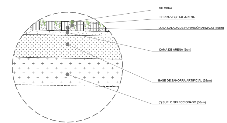
DETALLE NUEVO PAVICESPED SOBRE ZONA VERDE
