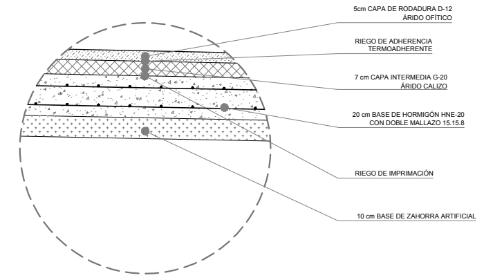
DETALLE NUEVA CALZADA SOBRE ACERA EXISTENTE E=1/25
