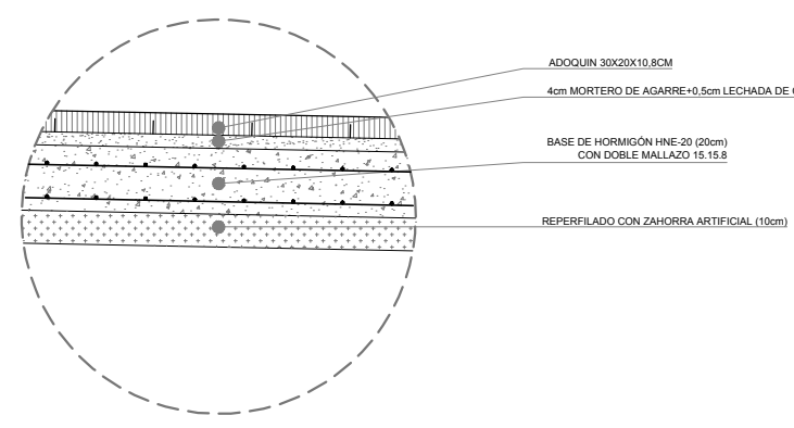
DETALLE DE CENEFA O PAVIMENTO CON ADOQUIN 30X20X10,8 EN CALZADA E=1/25
