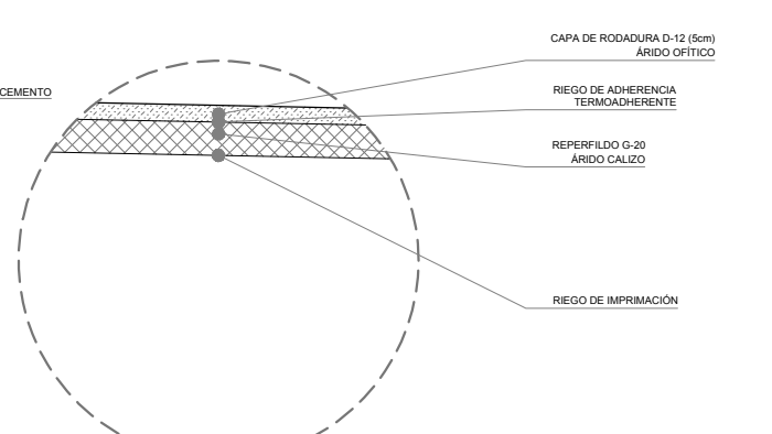
DETALLE NUEVO PARKING ASFALTO SOBRE AGLOMERADO EXISTENTE
