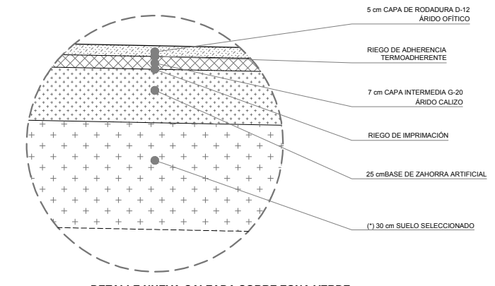
DETALLE NUEVA CALZADA SOBRE ZONA VERDE E=1/25
