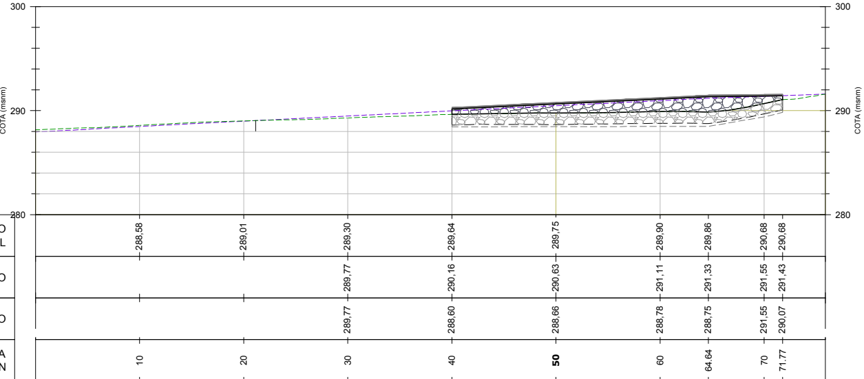
SECCIÓN ESCOLLERA MURO 2 Escala: 1/25
