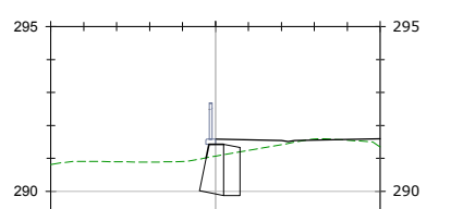
P.K.=0+071,77
