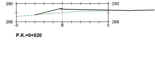
P.K.=0+020
