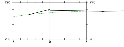
P.K.=0+010
