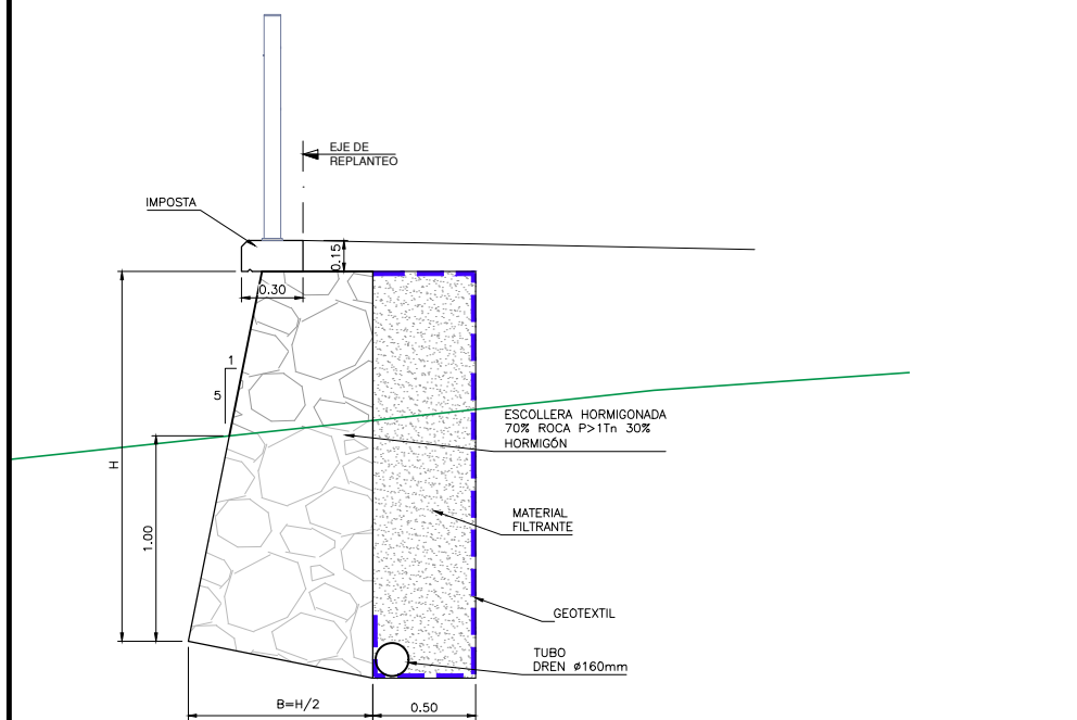
SECCIÓN ESCOLLERA MURO 2 Escala: 1/25
